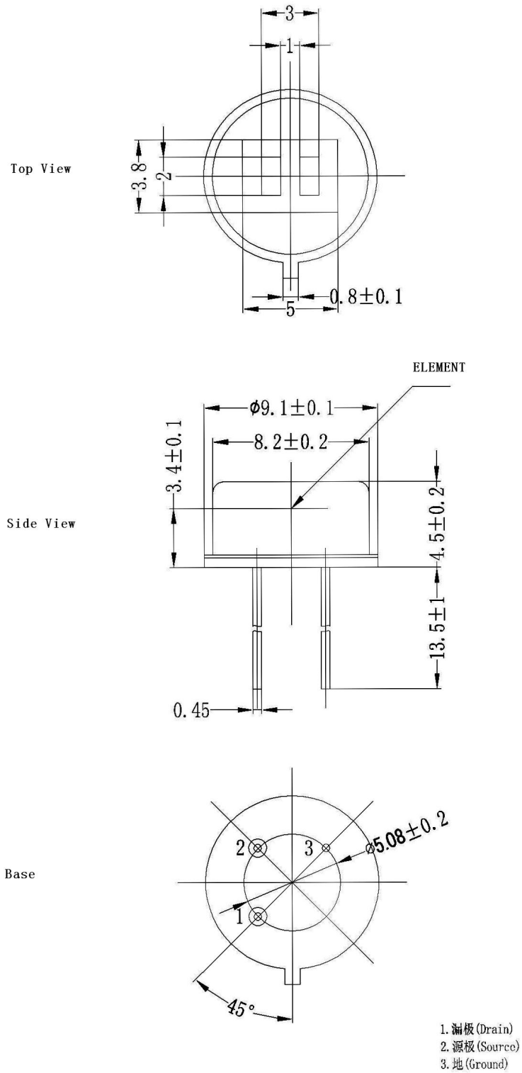
图 1 尺寸规格图
